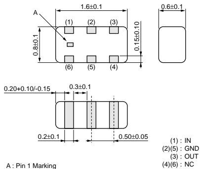
LFL18_TC1系列
